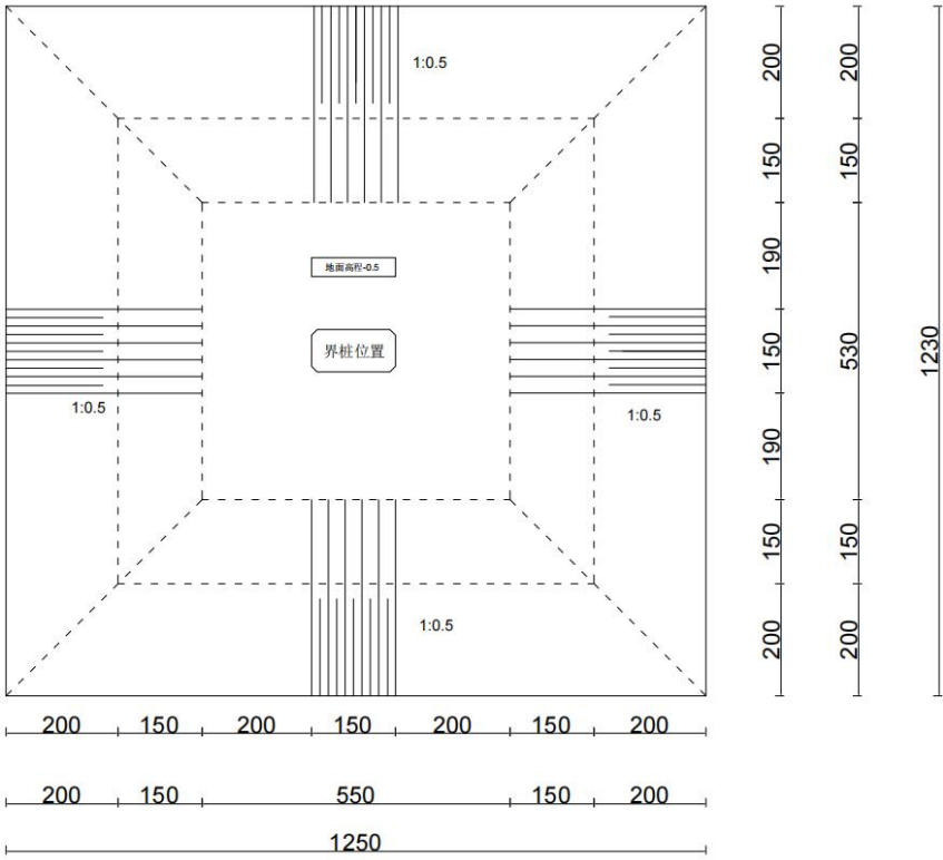
图 6.1-2 界桩结构图
