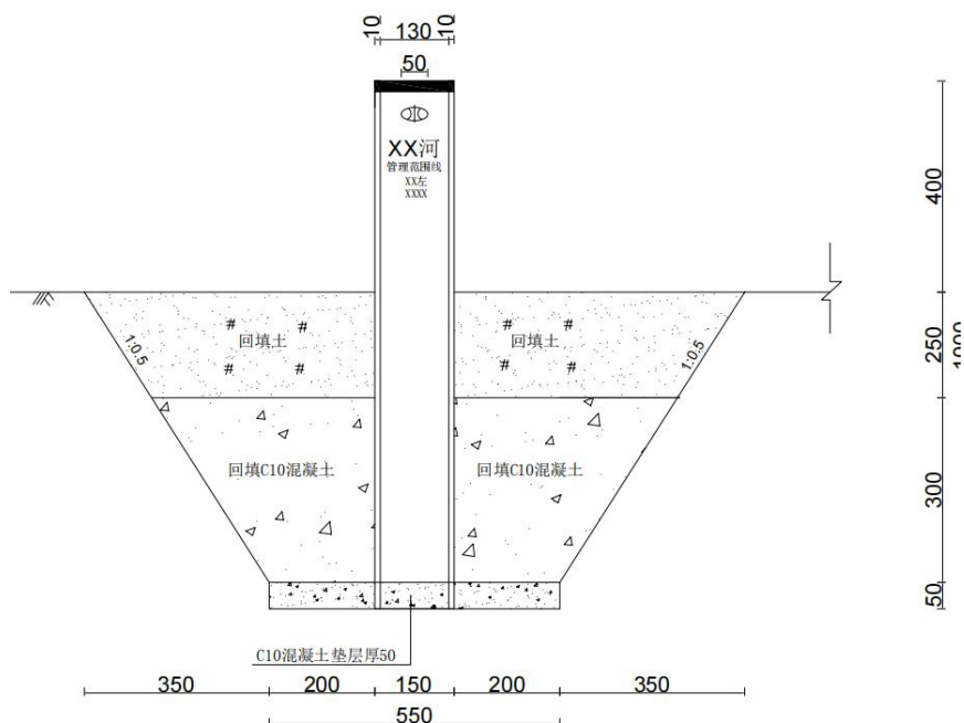
图 6.1-2 界桩结构图
