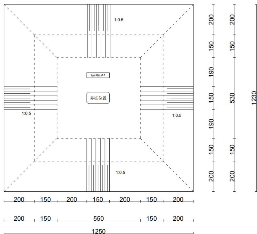
图 6.1-2 界桩结构图
