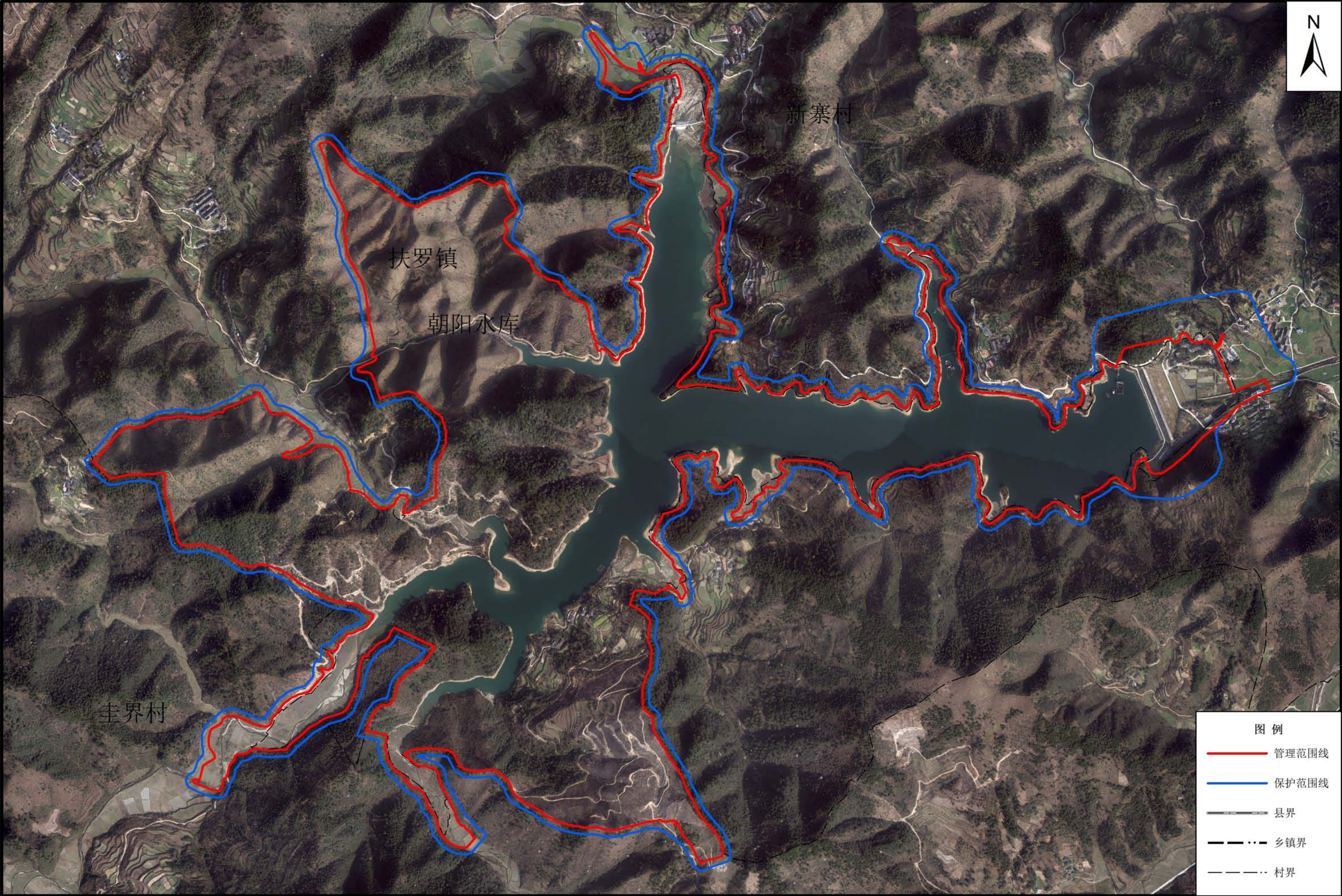
朝阳水库管理与保护范围划界成果示意图
