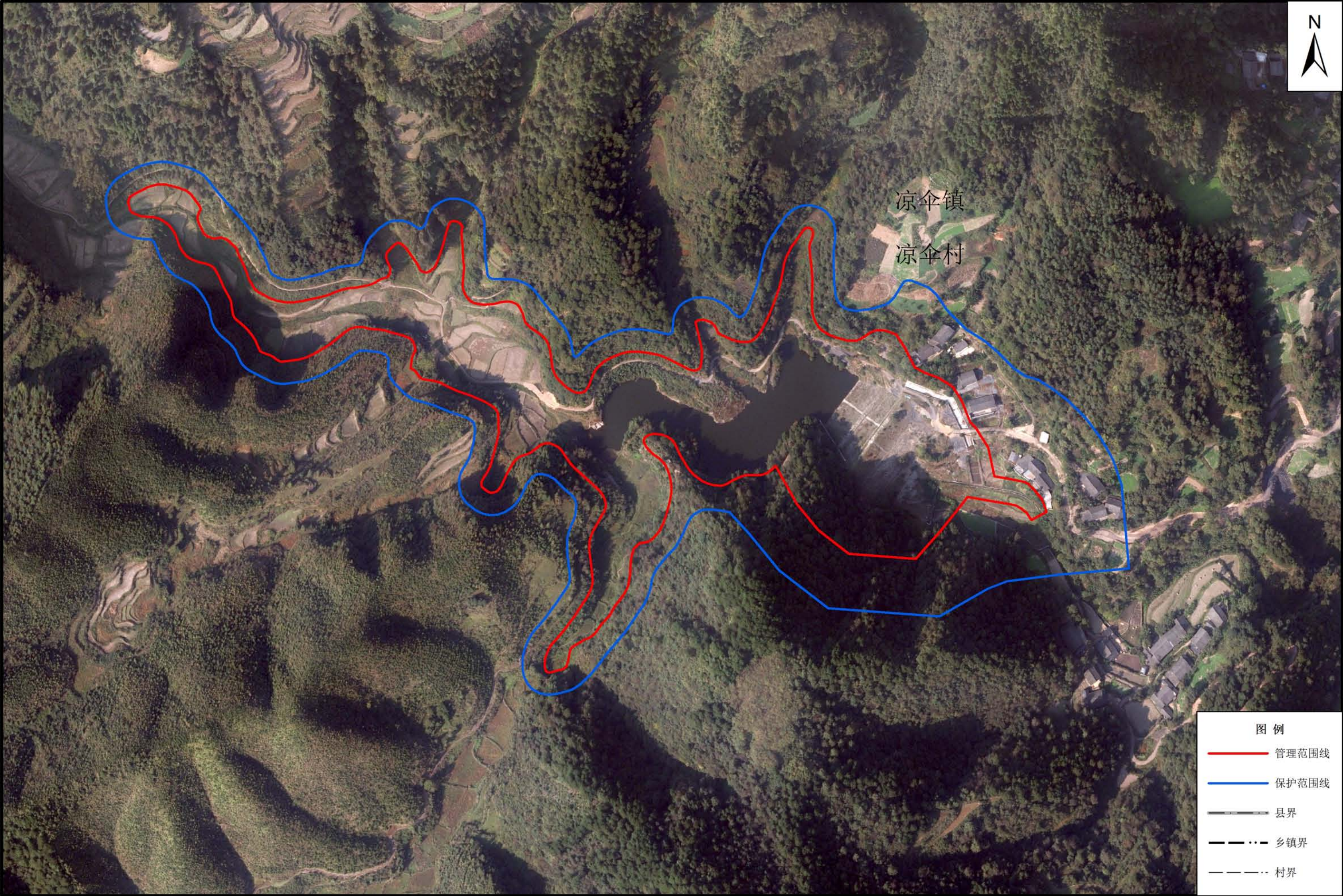
刘坪水库管理与保护范围划界成果示意图
